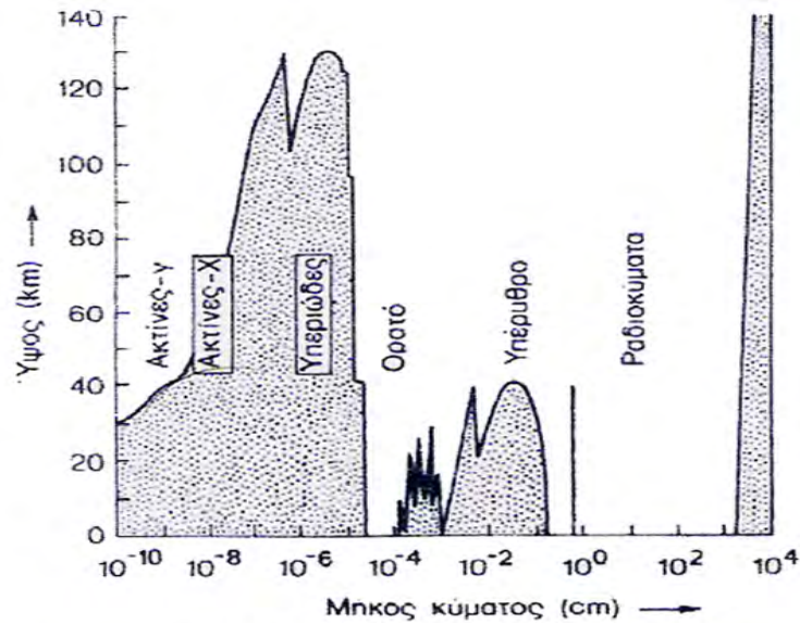
Το ηλεκτρομαγνητικό φάσμα και η απορρόφησή του στη γήινη ατμόσφαιρα.
